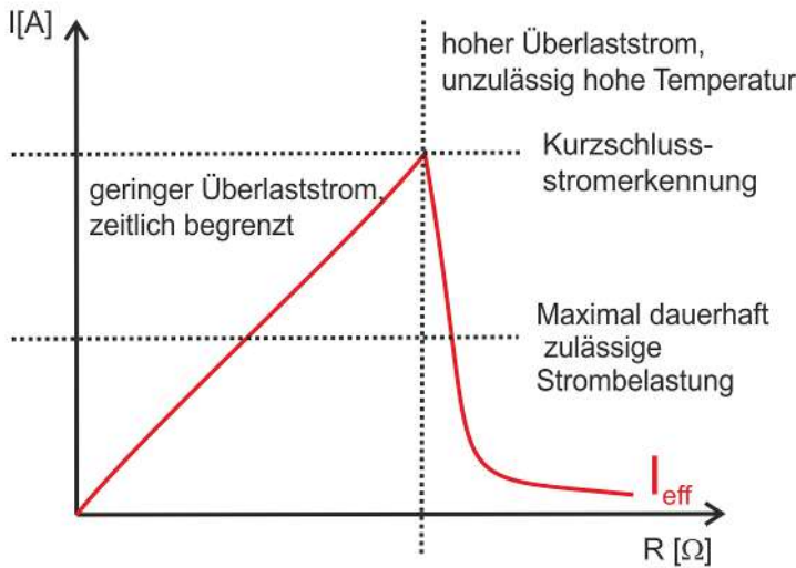
Abb. 8: Strombegrenzung bei Überlast
