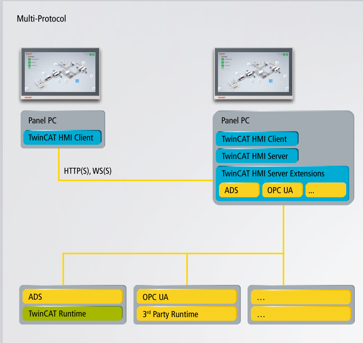
Der TwinCAT-HMI-Server kann mehrere Protokolle parallel verwenden.
