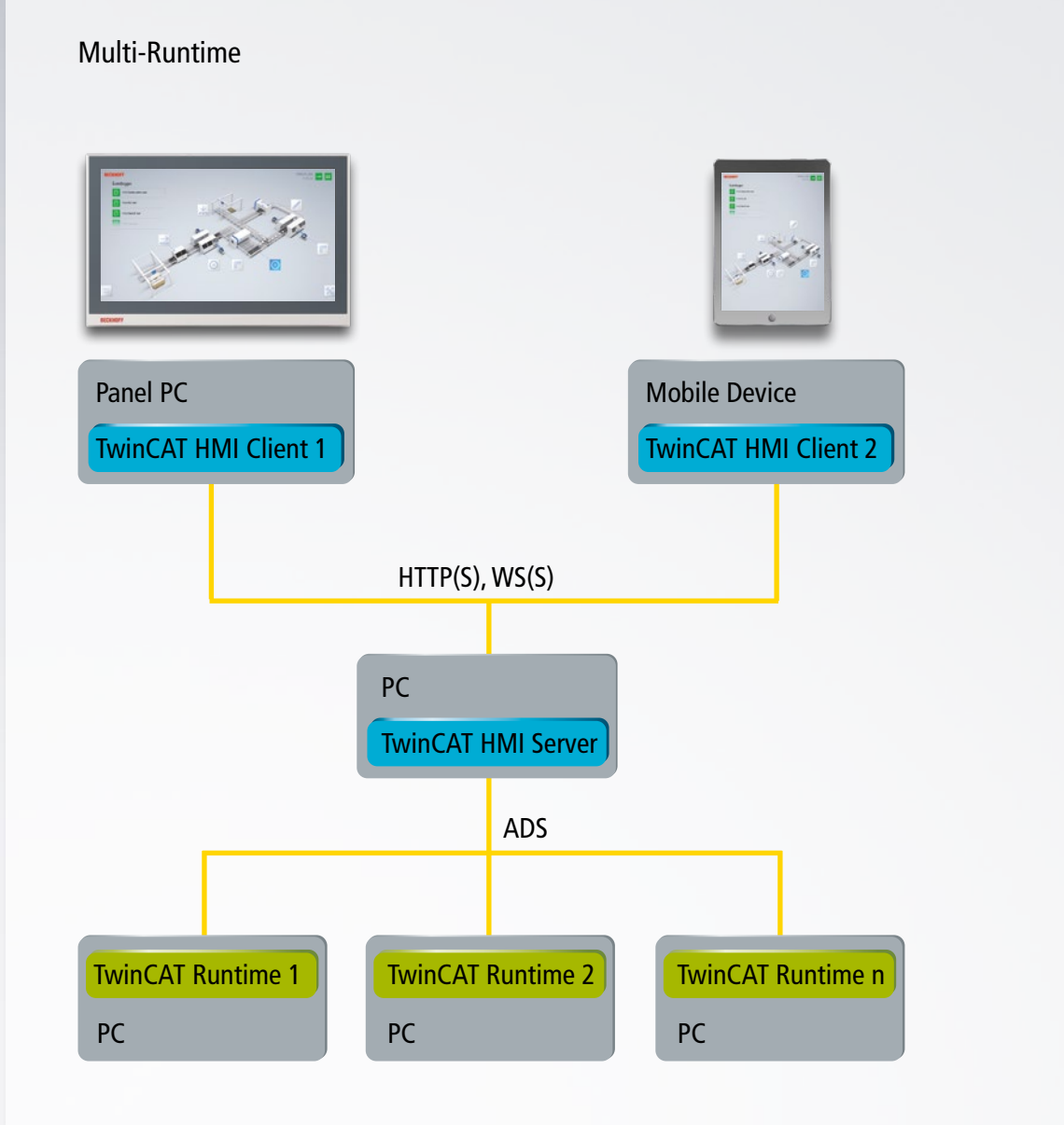
Der TwinCAT-HMI-Server unterstützt den Zugriff auf mehrere Runtime-Systeme.
