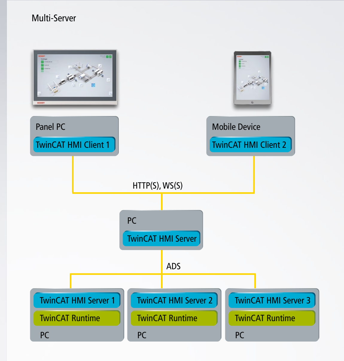
Ein Client kann parallel Daten von unterschiedlichen TwinCAT-HMI-Servern visualisieren.
