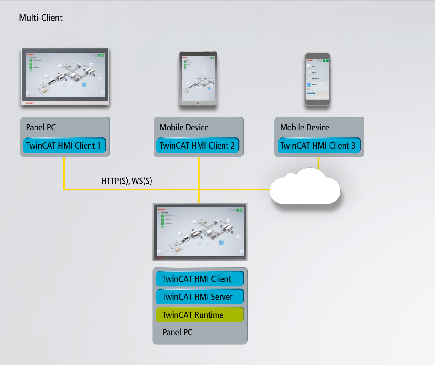
TwinCAT HMI kann von mehreren Clients parallel auf eine Runtime zugreifen und parallel bedient werden.
