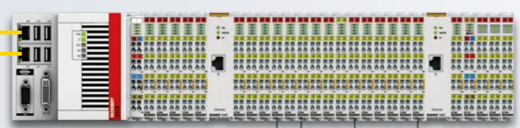
Embedded-PC, EtherCAT-Klemmen, Busklemmen
